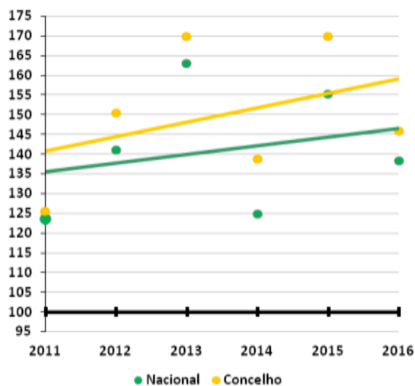
Figura 5.3.2.3.2 – Índices CIF e declives em Biologia e Geologia, às escalas Nacional e do Concelho, Ensino Secundário
